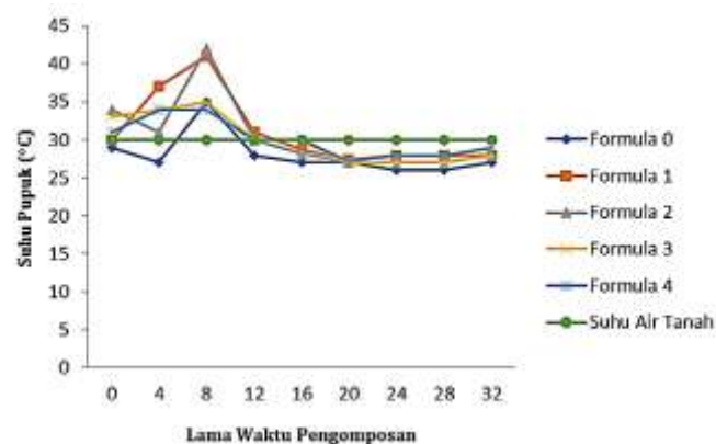
Gambar 1. Perubahan suhu pupuk pengomposan
