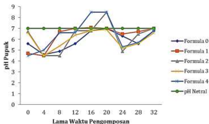
Gambar 2. pH pupuk organik pengomposan
